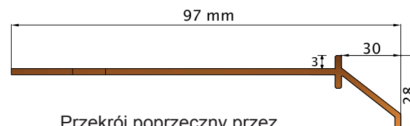
Przekrój poprzeczny przez profil BOLIX PAL-100
